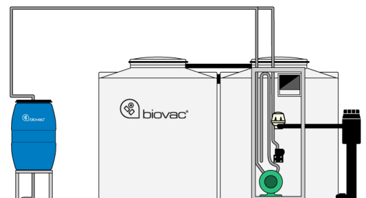
Tørt opstillet modtagertank
